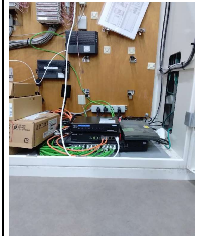
防災機器内 設置場所 (ONU, Si-R, SR-S)
