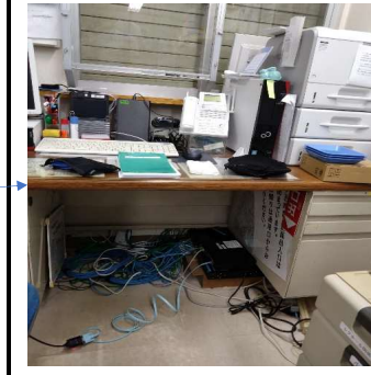
設置場所 (Si-R, SR-S) <カウンター下 床置き>
