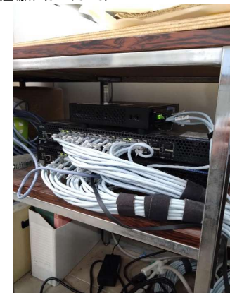
電話交換室ラック内(下段)
