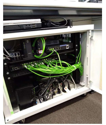
ラックの中に集約 機器設置場所 (Si-R, SR-S, SH)
